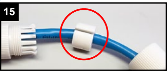
15 Kabel durch den seitlichen Schlitz in die Dichtung pressen.
