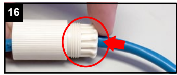
16 Dichtung in den Schraubbolzen pressen.
