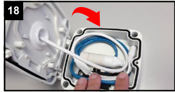
18 Verkabelung vollständig in die Box legen und Deckel schließen.
