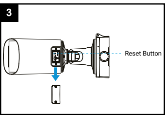
3 Für Reset: Fünf Sekunden lang die Taste gedrückt halten.
