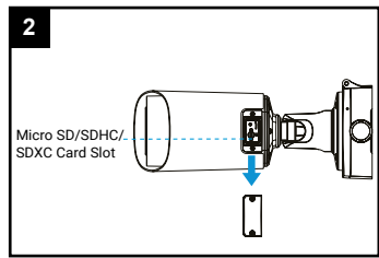
2 Derunter befindet sich ein Kartenslot. Dieser ist je nach Modellvariante für microSD Speicherkarten oder für Nano SIM
